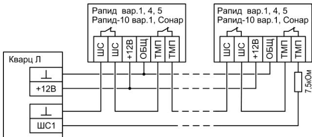
Рис.А7 Схема подключения охранных извещателей Рапид вар.1,4,5, Рапид-10 вар.1, Сонар
