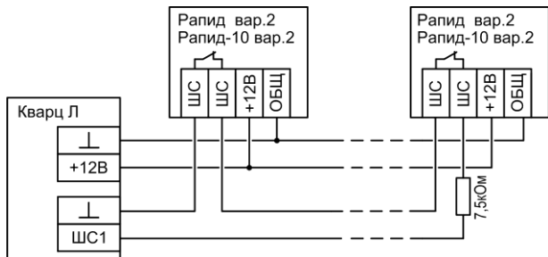
Рис.А6 Схема подключения охранных извещателей Рапид вар.2, Рапид-10 вар.2
